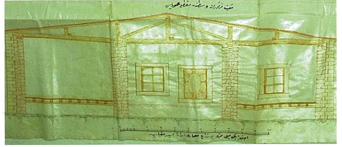
Fotoğraf 1b: Kayseri İdadisinin Başbakanlık Osmanlı Arşivinde bulunan cephe çizimi.
