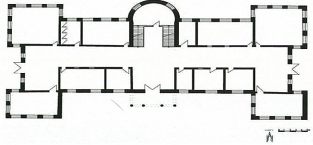
Plân 1: Kayseri İdadisi (Lisesi) birinci kat plânı.
